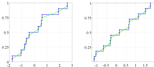
Figure – Fréquences cumulées (en bleue) et de fonction de répartition empirique (courbe verte) pour 11 observations (à droite).
